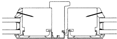
ASTRAGAL STILE
